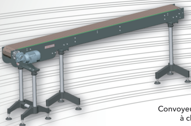
Convoyeur droit à chaîne à palette.
